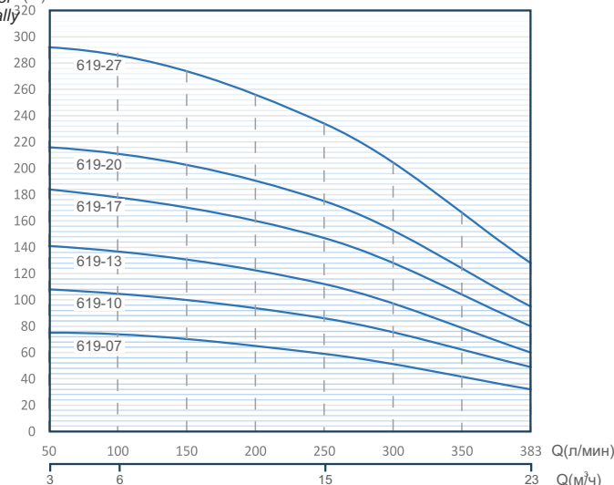
Характеристики насоса згідно з ISO 9906
