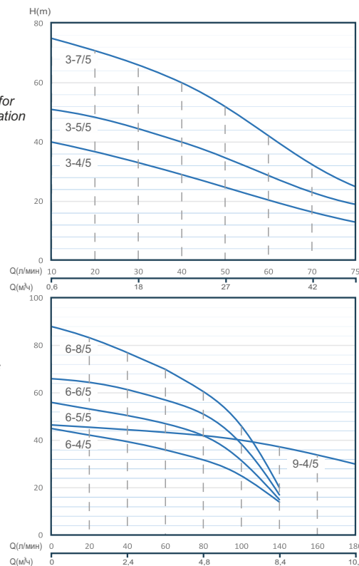
Характеристики насоса згідно з ISO 9906
