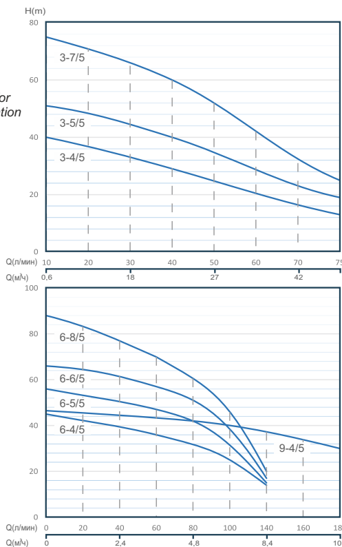
Характеристики насоса згідно з ISO 9906
