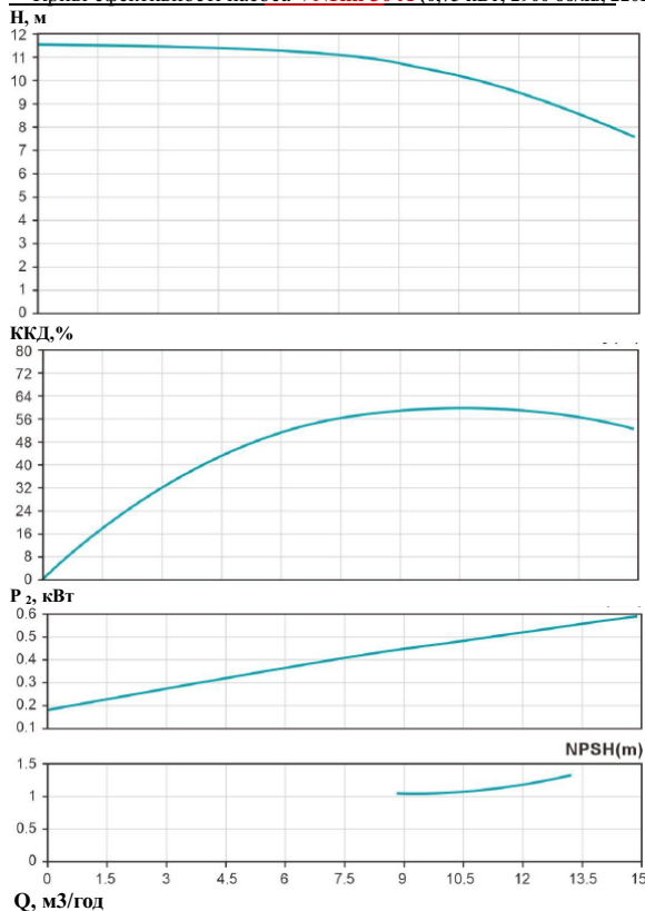
Криві ефективності насоса VNRm 50 (1,1 кВт; 2900 об/хв, 220 В)
