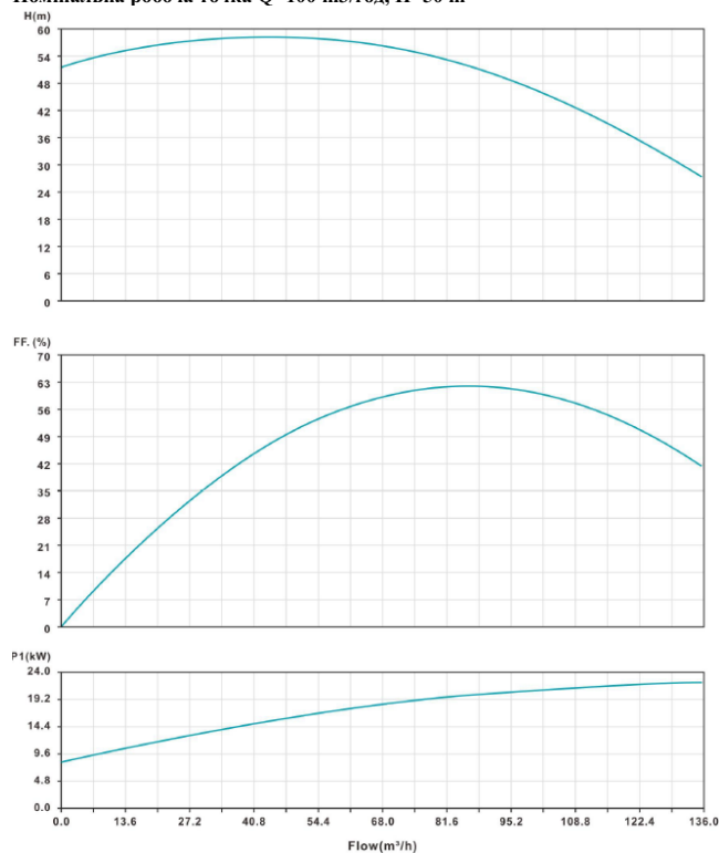
Криві ефективності насоса VNR 80-200 (22,0 кВт; 2900 об/хв, 380В) Номінальна робоча точка Q=100 \text{ м}^3/\text{год} , H=50 \text{ м}
