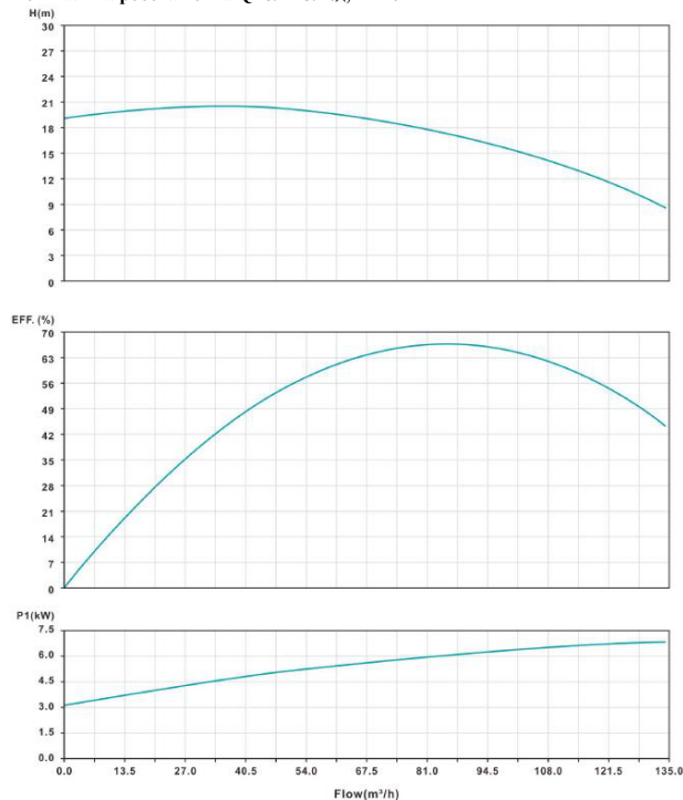
Криві ефективності насоса VNR 80-125 A (7,5 кВт; 2900 об/хв, 380В) Номінальна робоча точка Q=89 м³/год, H=16 м
