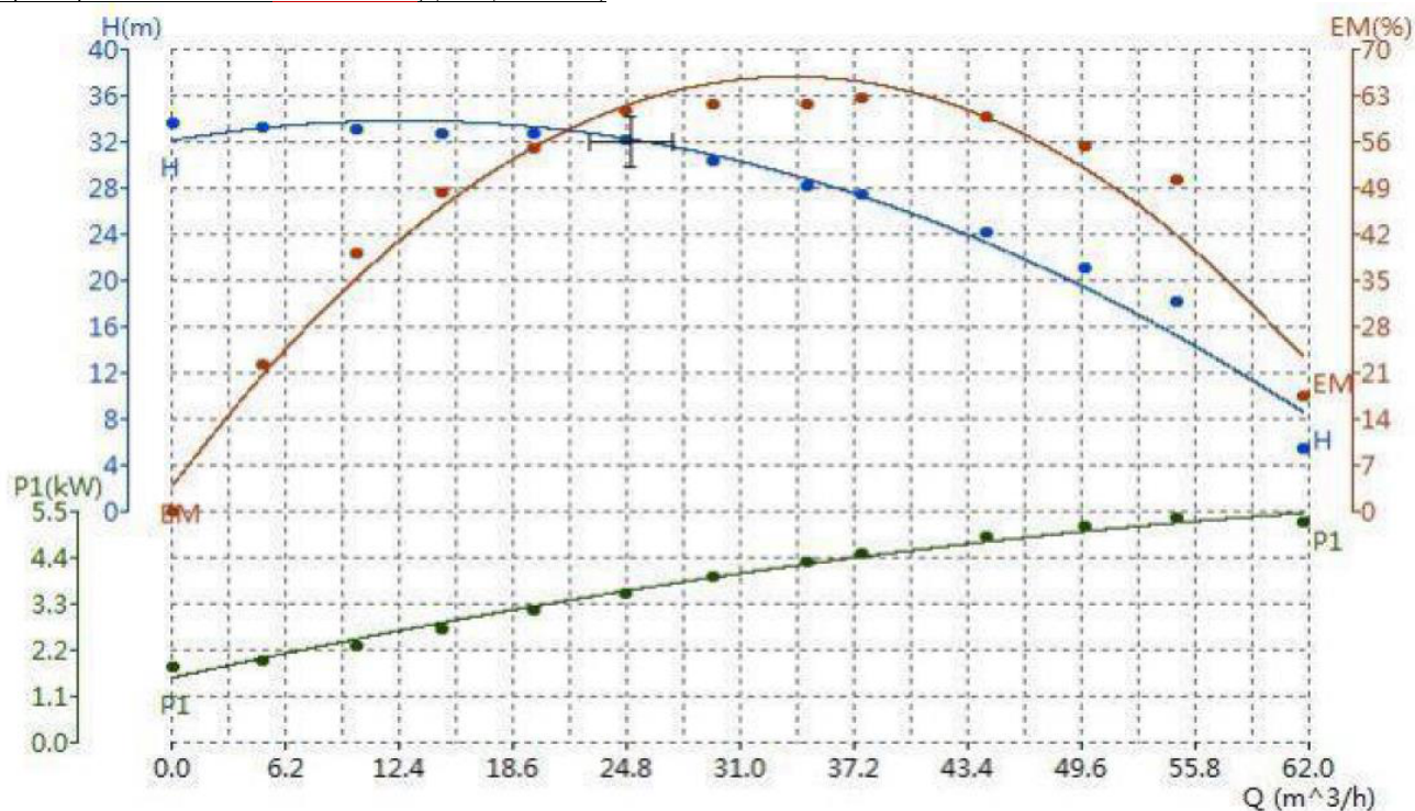
Криві ефективності насоса VNR 50 – 200 (7,5 кВт; 2900 об/хв)
