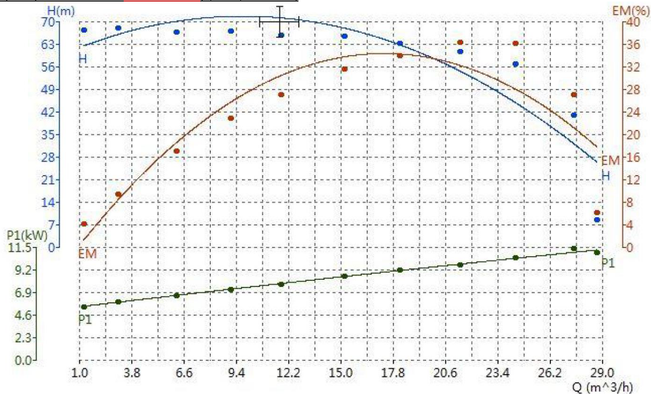
Криві ефективності насоса VNR 40 – 250 А (7,5 кВт; 2900 об/хВ)
