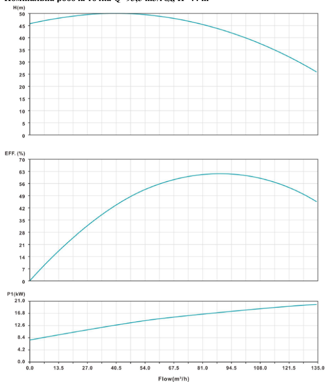
Криві ефективності насоса VNR 80-200 A (18,5 кВт; 2900 об/хв, 380В) Номінальна робоча точка Q=93,5 \text{ м}^3/\text{год} , H=44 \text{ м}
