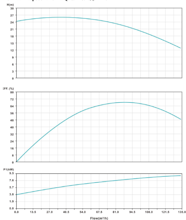
Криві ефективності насоса VNR 80-125 (11,0 кВт; 2900 об/хв, 380В) Номінальна робоча точка Q=89 м³/год, H=16 м
