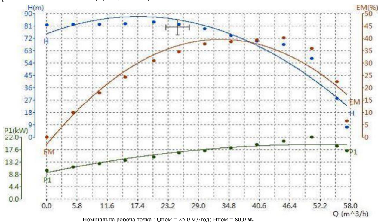
Криві ефективності насоса VNR 50 – 250 (15,0 кВт; 2900 об/хв)
