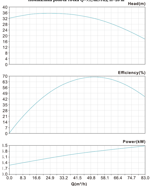
Криві ефективності насоса VNR 80-160 Б (7,5 кВт; 2900 об/хв, 380В) Номінальна робоча точка Q=93,5 \text{ м}^3/\text{год} , H=28 \text{ м}
