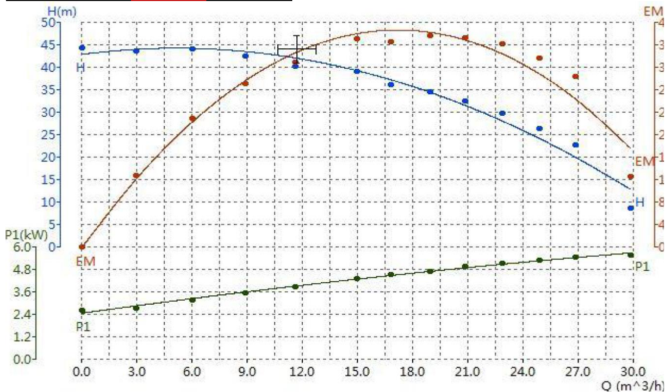
Криві ефективності насоса VNR 50 – 200 В (4,0 кВт; 2900 об/хв)
