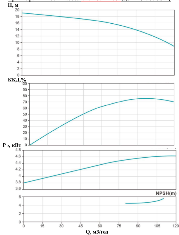
Криві ефективності насоса VNR 80 – 100 (5,5 кВт; 2900 об/хв)
