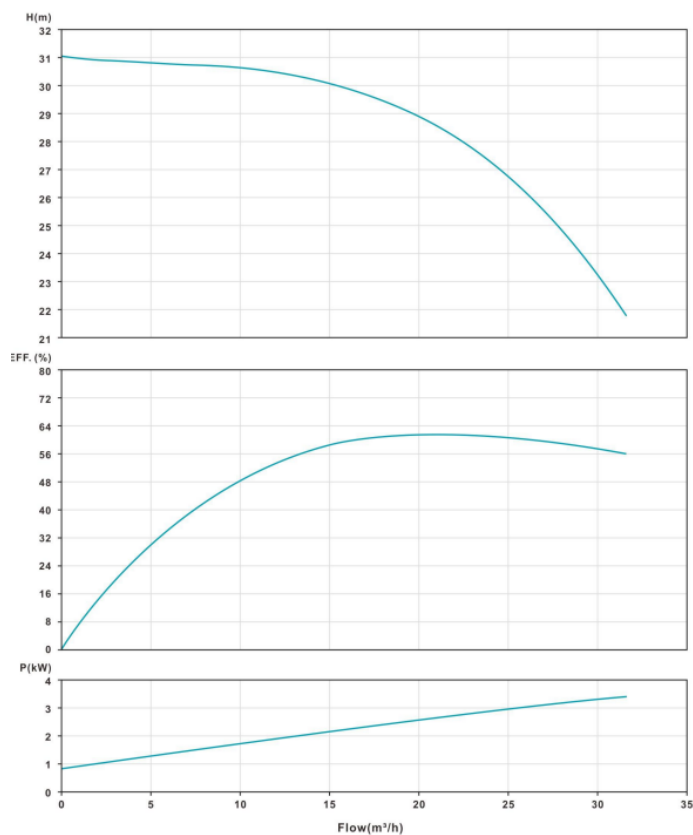
Криві ефективності насоса VNR 50 – 160 A (3,0 кВт; 2900 об/хВ)
