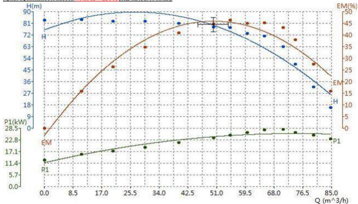
Криві ефективності насоса VNR 65 – 250 A (18,5 кВт; 2900 об/хв).
