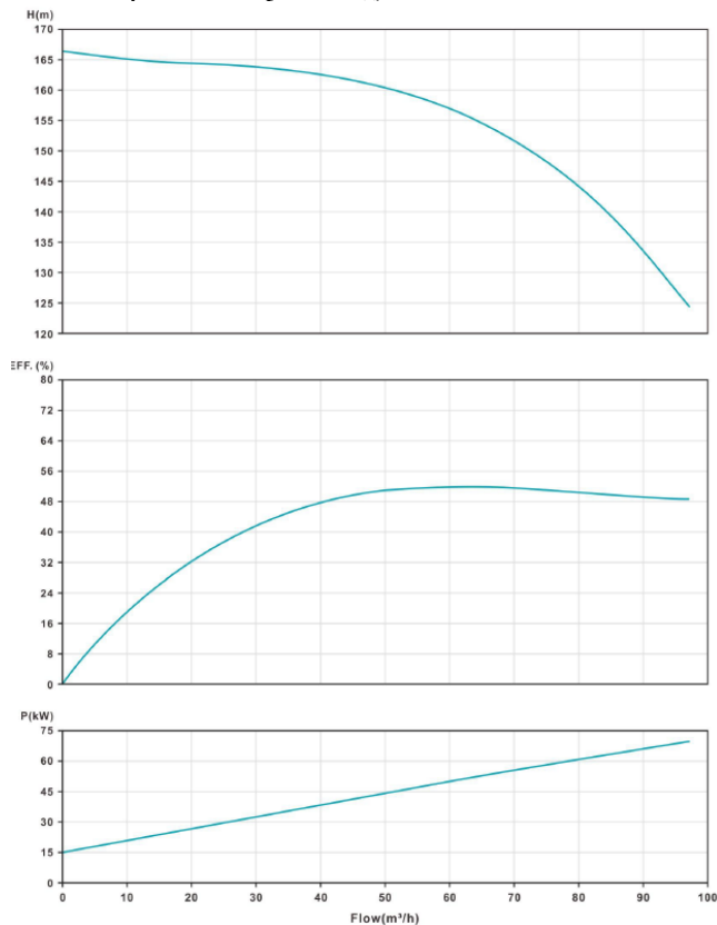
Криві ефективності насоса VNR 80-350 (75,0 кВт; 2900 об/хв) Номинальна робоча точка Q=72 \text{ м}^3/\text{год} , H=150 \text{ м}
