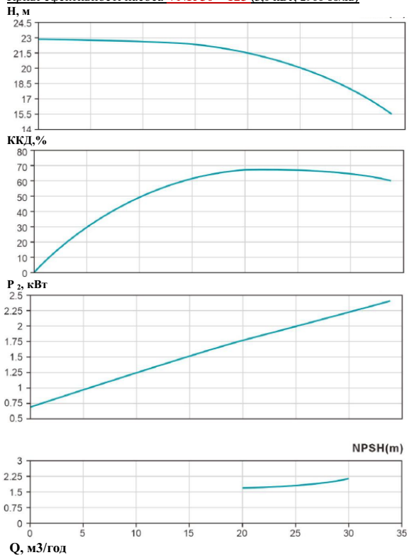
Криві ефективності насоса VNR 50 – 125 (3,0 кВт; 2900 об/хв)
