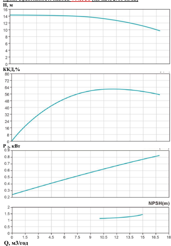
Криві ефективності насоса VNR 50 (1,1 кВт; 2900 об/хв)
