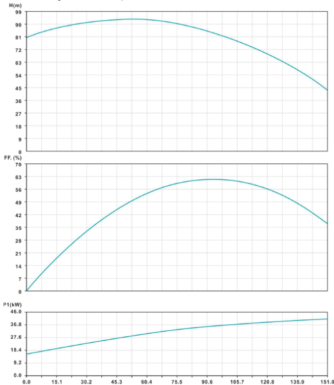
Криві ефективності насоса VNR 80-250 B (37,0 кВт; 2900 об/хв, 380В)
