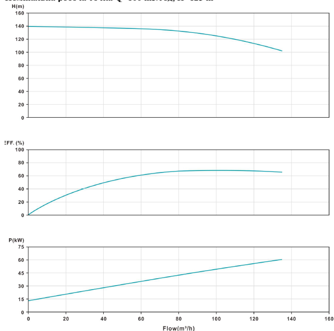
Криві ефективності насоса VNR 80-315 (75,0 кВт; 2900 об/хв, 380В) Номинальна робоча точка Q=100 \text{ м}^3/\text{год} , H=125 \text{ м}
