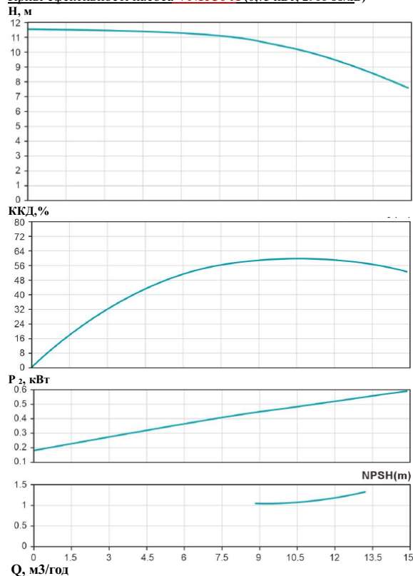
Криві ефективності насоса VNR 50 (1,1 кВт; 2900 об/хв)
