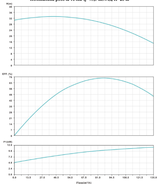
Криві ефективності насоса VNR 80-160 A (11,0 кВт; 2900 об/хв, 380В) Номінальна робоча точка Q=93,5 \text{ м}^3/\text{год} , H=28 \text{ м}
