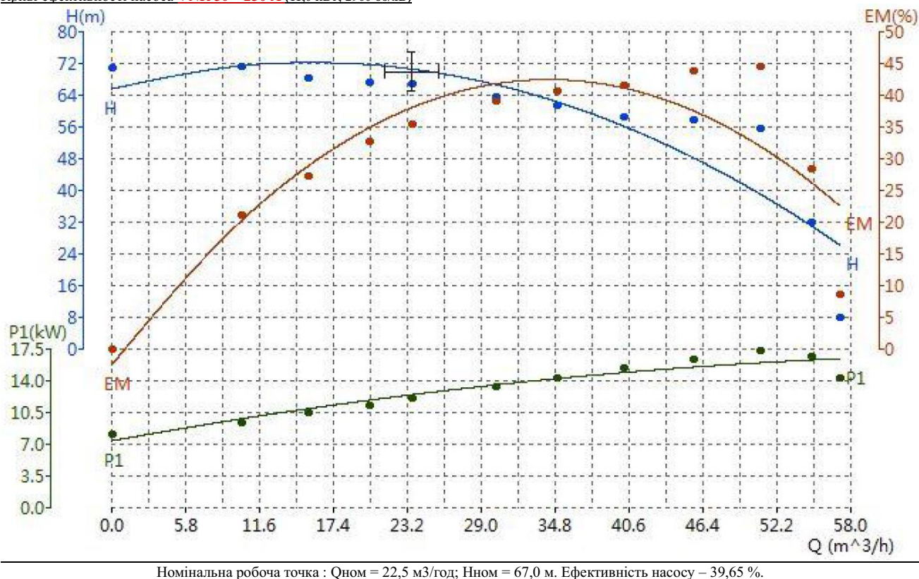
Криві ефективності насоса VNR 50 – 250 A (11,0 кВт; 2900 об/хв)
