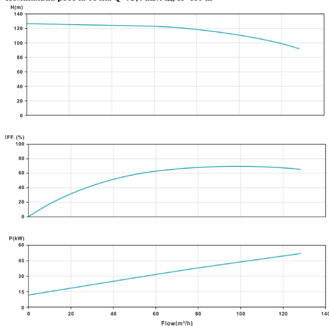
Криві ефективності насоса VNR 80-315 A (55,0 кВт; 2900 об/хв, 380В) Номинальна робоча точка Q=93,4 \text{ м}^3/\text{год} , H=110 \text{ м}
