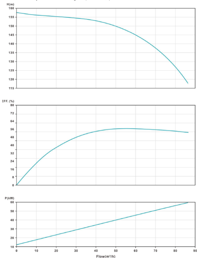
Криві ефективності насоса VNR 80-350 A (55,0 кВт; 2900 об/хв) Номинальна робоча точка Q=64,0 \text{ м}^3/\text{год} , H=142 \text{ м}
