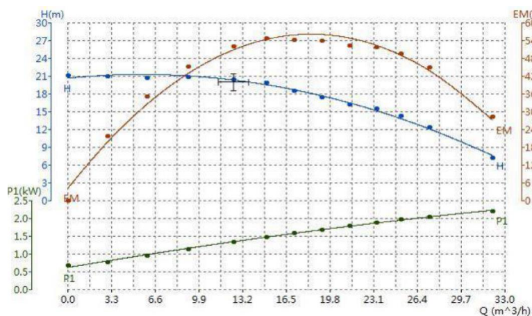
Криві ефективності насоса VNR 40 – 125 (1.5 кВт; 2900 об/хв)
